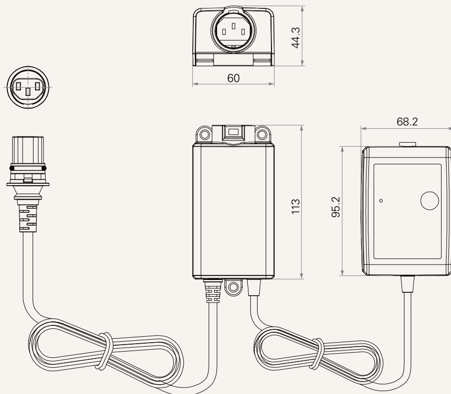
TEB2連接到控制盒之AC線
